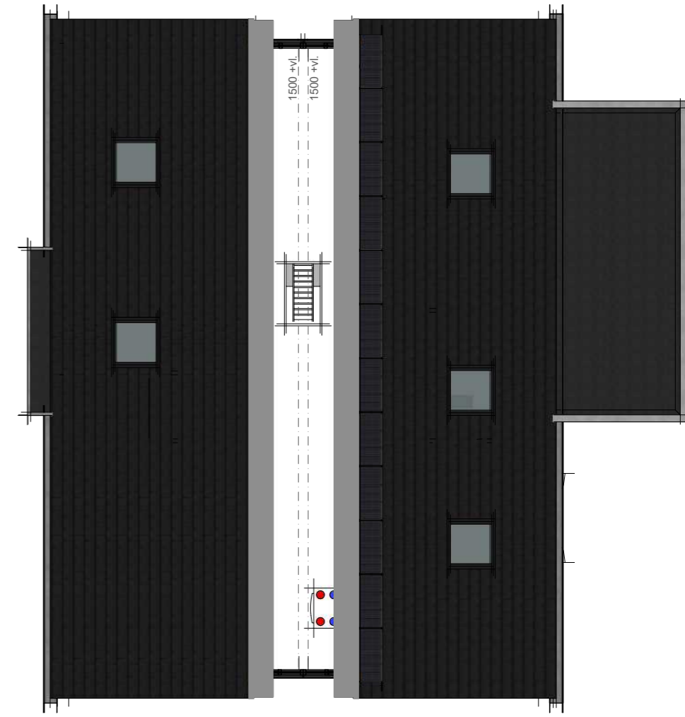
zolder / 2de verdieping
